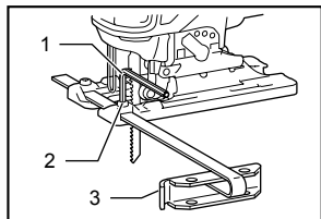
1. Clé hexagonale 2. Boulon 3. Guide de garde
