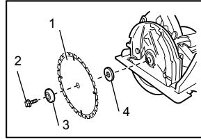
1. Lame 2. Boulon hexagonal 3. Bague externe 4. Flasque intérieur
